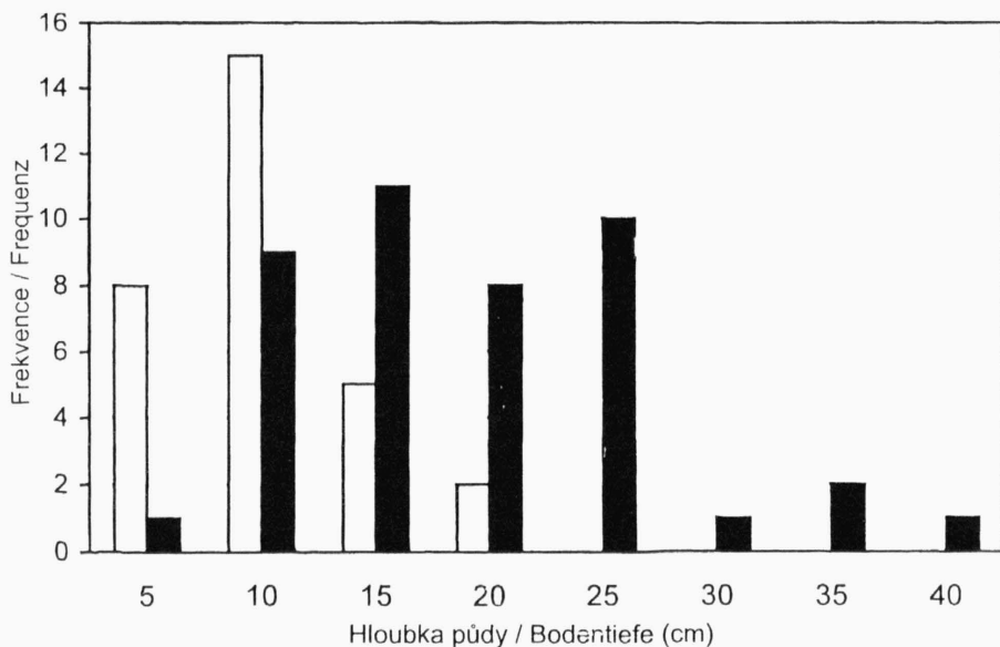
Obr. 5. – Srovnání hĺbky pŕdy pod trsy Stipa eriocalis (bílé sloupce) a S. pulcherrima (černé sloupce). Data pro S. eriocalis jsou ze Svatého kopečku, pro S. pulcherrima ze Svatého kopečku, Soutěšky a Kotelné. Kategorie hĺbky pŕdy jsou po 5 cm.
