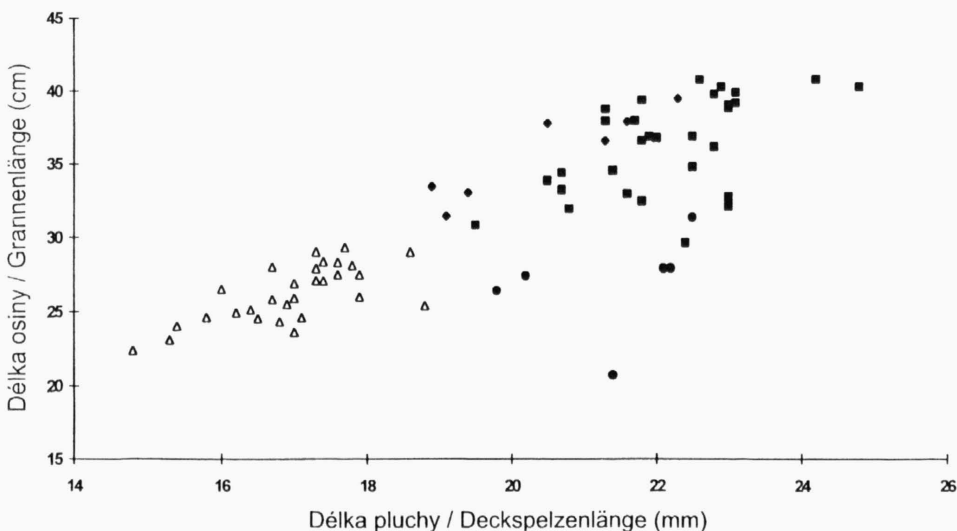
Obr. 4. – Délka pluchy v poměru k délce osiny u Stipa eriocaulis (Δ) a S. pulcherrima (● – Svatý kopeček, ■ – Soutěška, ◆ – Kotelná).
