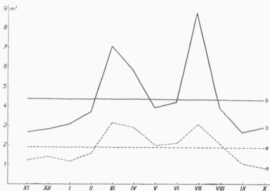
Abb. 2. — Die Abflussverhältnisse des Blanice-Flusses: Die mittleren monatlichen Abflussmengen in m³/s in dem Zeitraume der Jahre 1951—1960. — a: Pegel Podedvory, b: Pegel Heřmaň (s. Längsprofil des Flusses).
