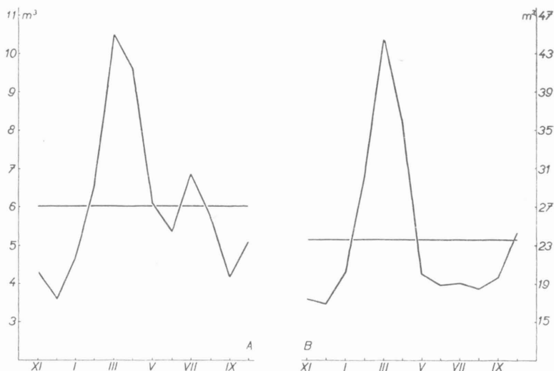
Abb. 1. — Die Abflussverhältnisse des Lužnice-Flusses: Die mittleren monatlichen Abflussmengen in m³/s in dem Zeitraume der Jahre 1931—1960. — A: Pegel Pilař, B: Pegel Bechyně (s. Längsprofil des Flusses).
