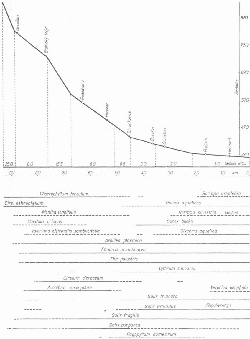
Abb. 4. — Längsprofil der Blanice (von der Quelle bis zur Mündung) mit Verbreitungslinien einiger Uferpflanzen.
